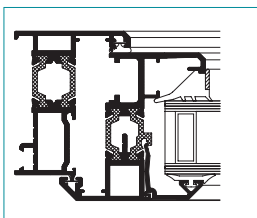
Jamb
