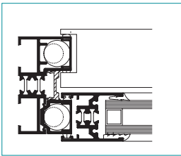
VSW jamb
